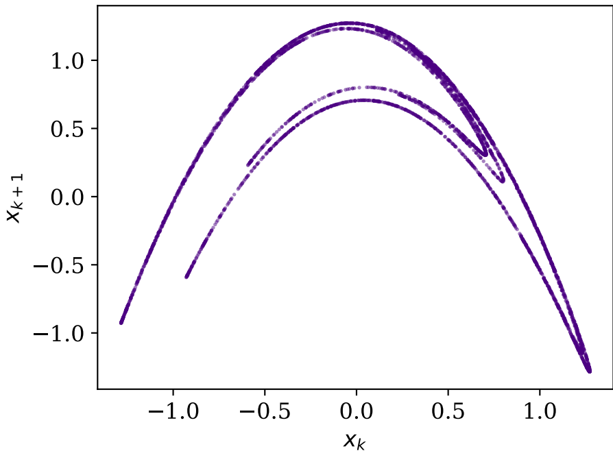
Диаграмма возвратов ( x_{k+1} от x_k )
